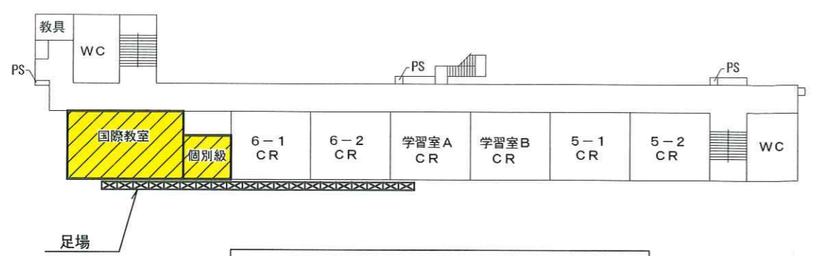
4階 平面図 S=1/600
