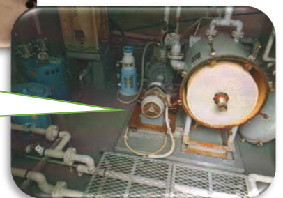
プール循環機室 床防水塗装工事 (屋上循環機室)
