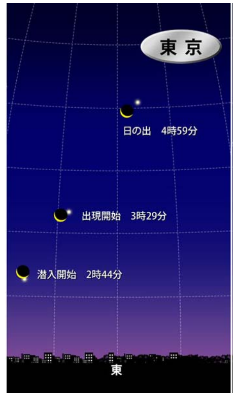
金星食：国立天文台HPより
